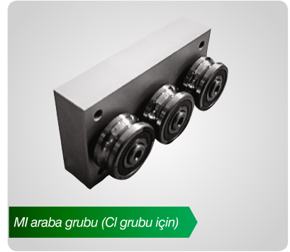
WINMAN Lineer Aktüatör
