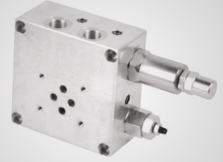
WINMAN modüler tandem sıfırlama valfi
